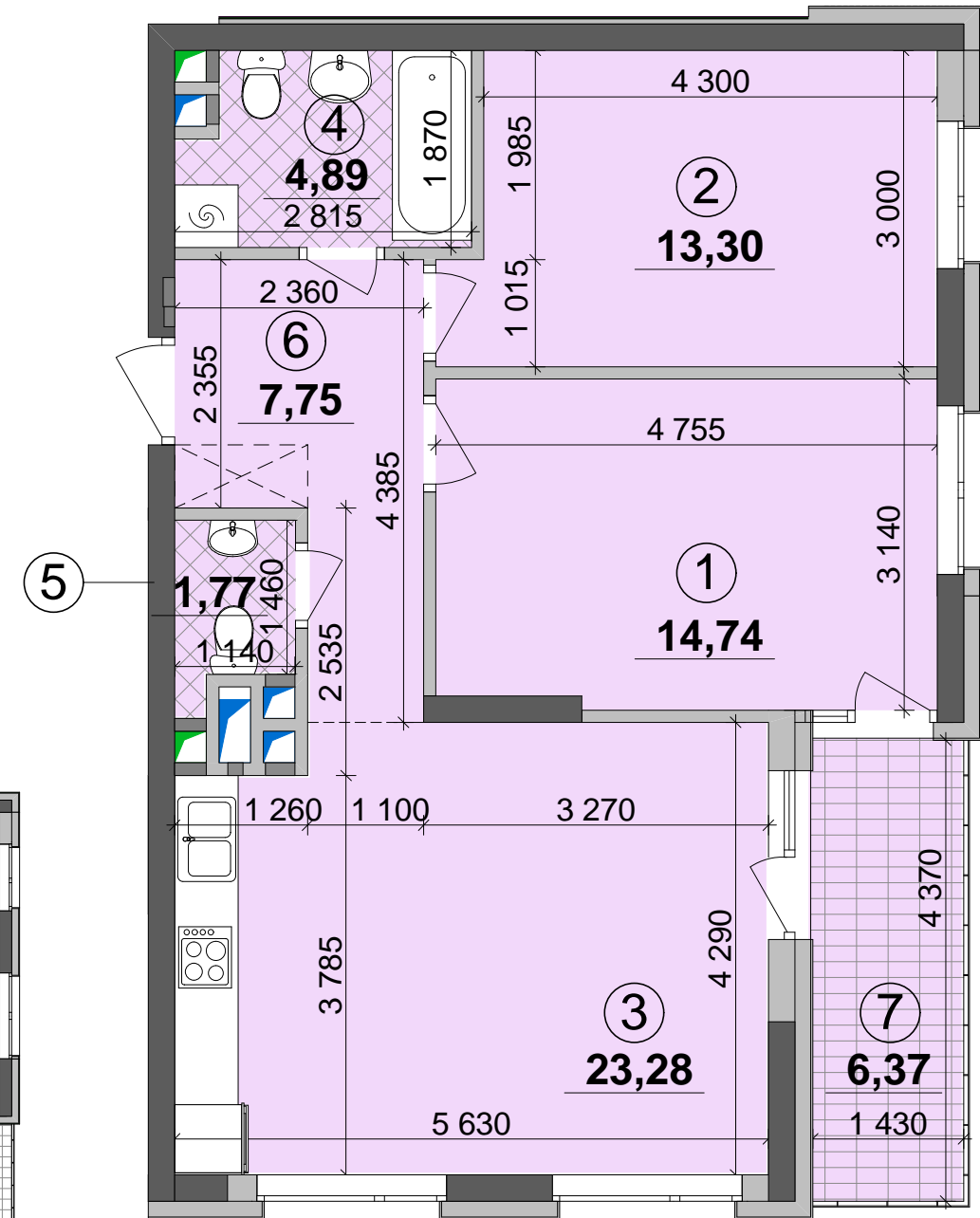
План квартири без перегородок
