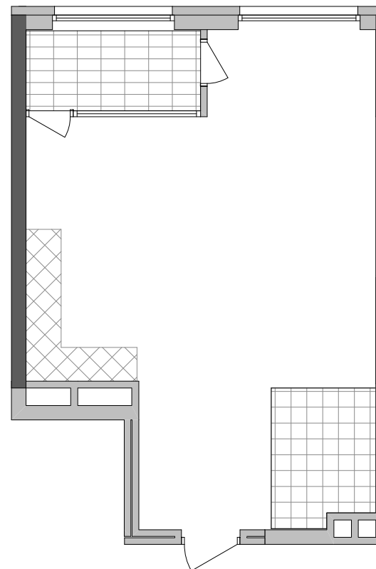
План квартири без перегородок
